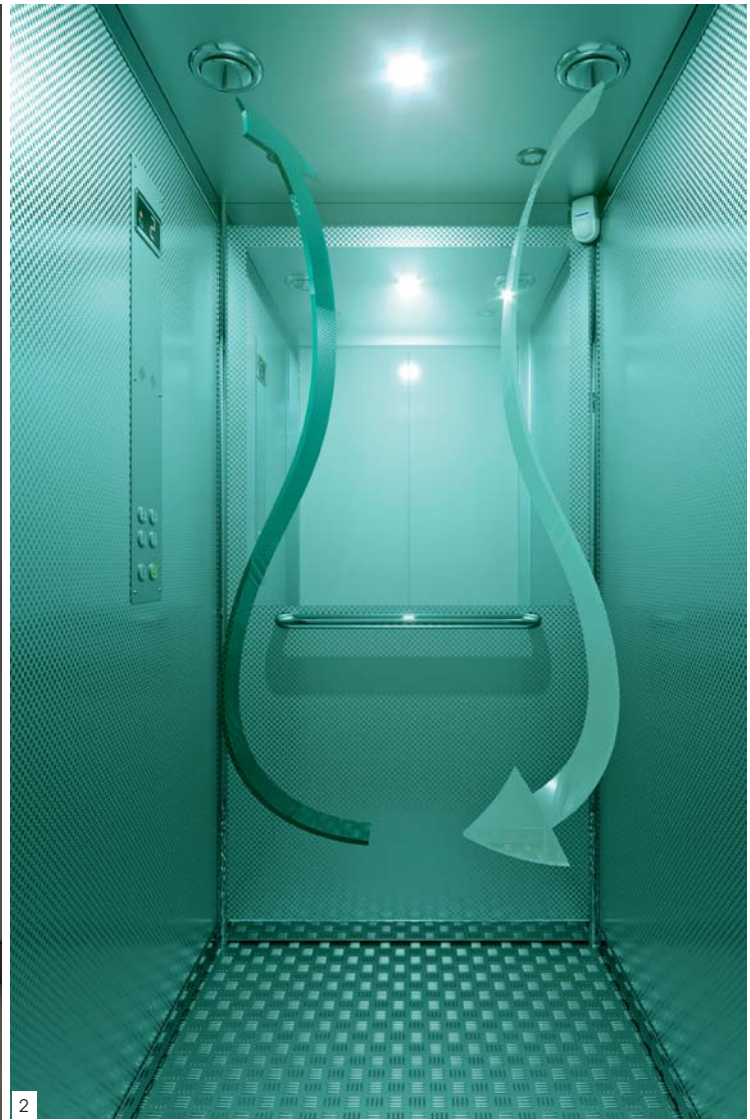
1. Cabina Sky Lift, studio MaMa Design: un lucernario ellissoidale ricrea la sensazione visiva del cielo e del sole con un'illuminazione che varia nel corso della giornata 2. CARE: schema del flusso di ventilazione con filtro assoluto HEPA Immagini courtesy IGV Group
